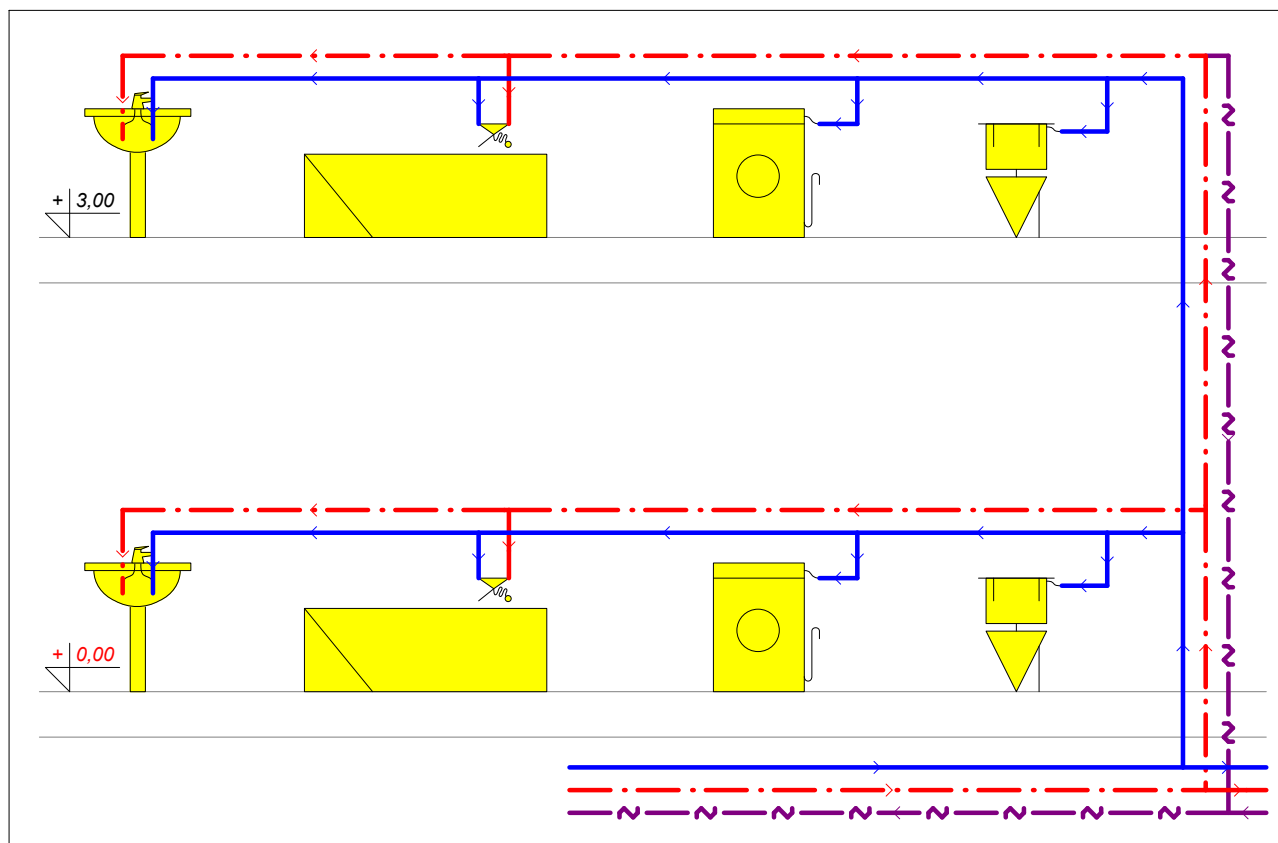
Fragment rozwinięcia z narysowaną siecią przewodów
