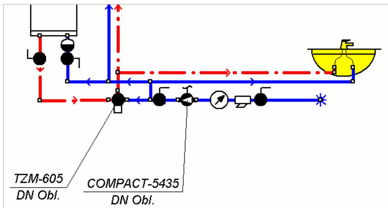
Przykład podłączenia zaworu mieszającego oraz regulatora ciśnienia
