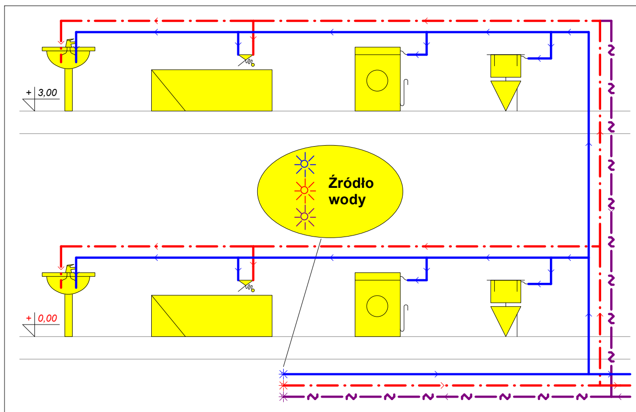
Fragment rysunku ze źródłem wody i siecią przewodów rozprowadzających
