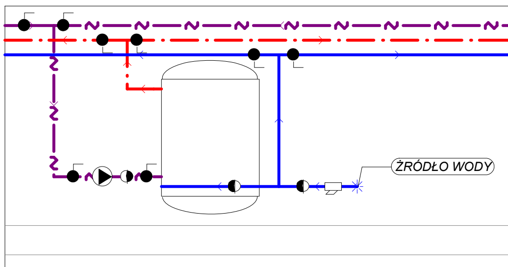
Fragment rozwinięcia z narysowanymi kształtkami i armaturą
