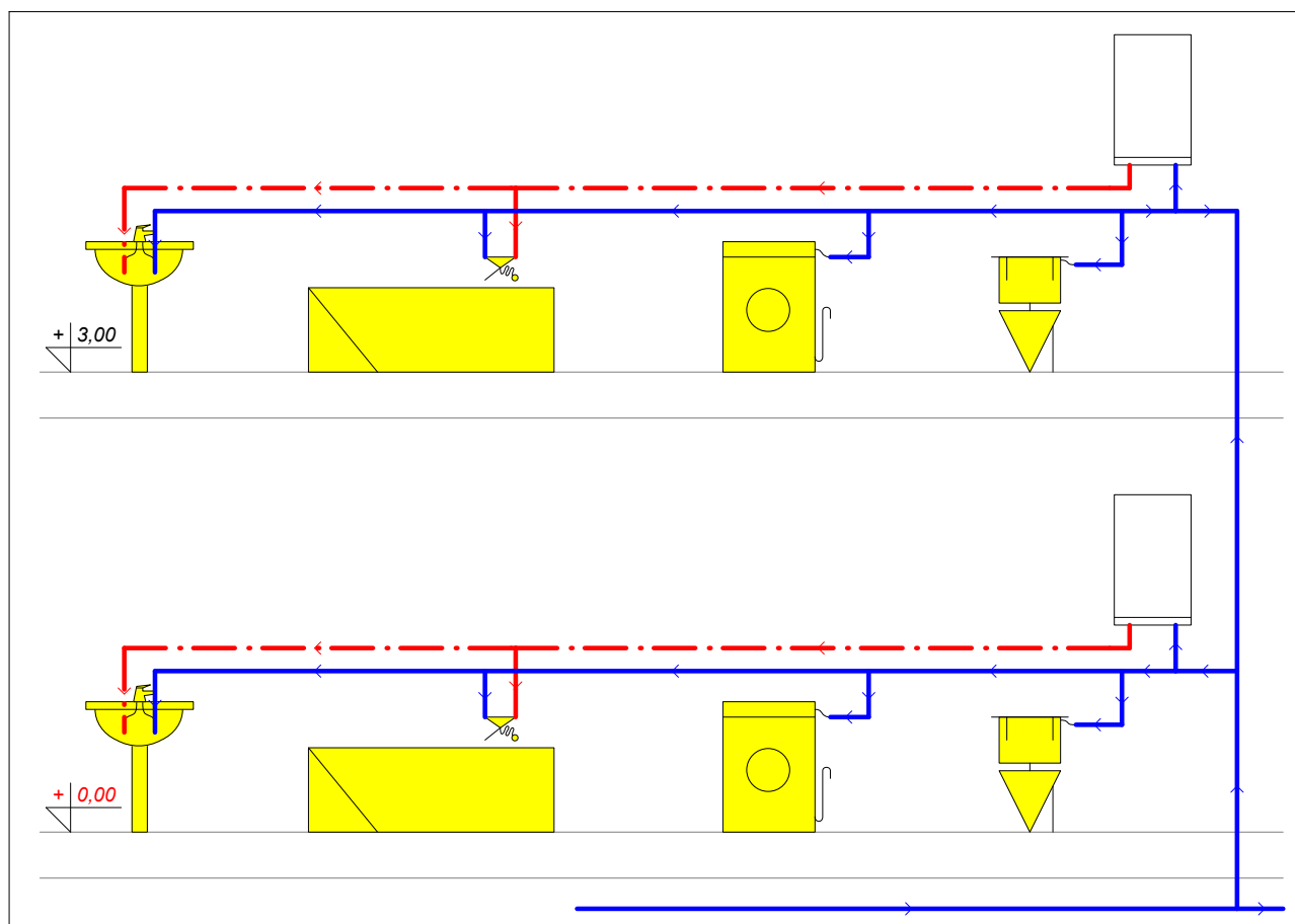
Fragment instalacji z indywidualnymi podgrzewaczami wody
