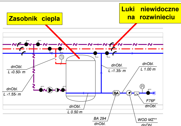
Fragment rozwinięcia z dorysowanymi przewodami rozprowadzającymi, zasobnikiem ciepła, dodatkowymi urządzeniami i niewidocznymi łukami
