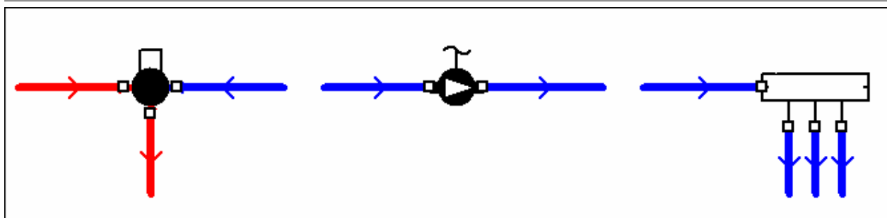
Przykłady połączeń rozdzielaczy, termostatyczny zaworów mieszających do CWU oraz zaworów regulujących ciśnienie
