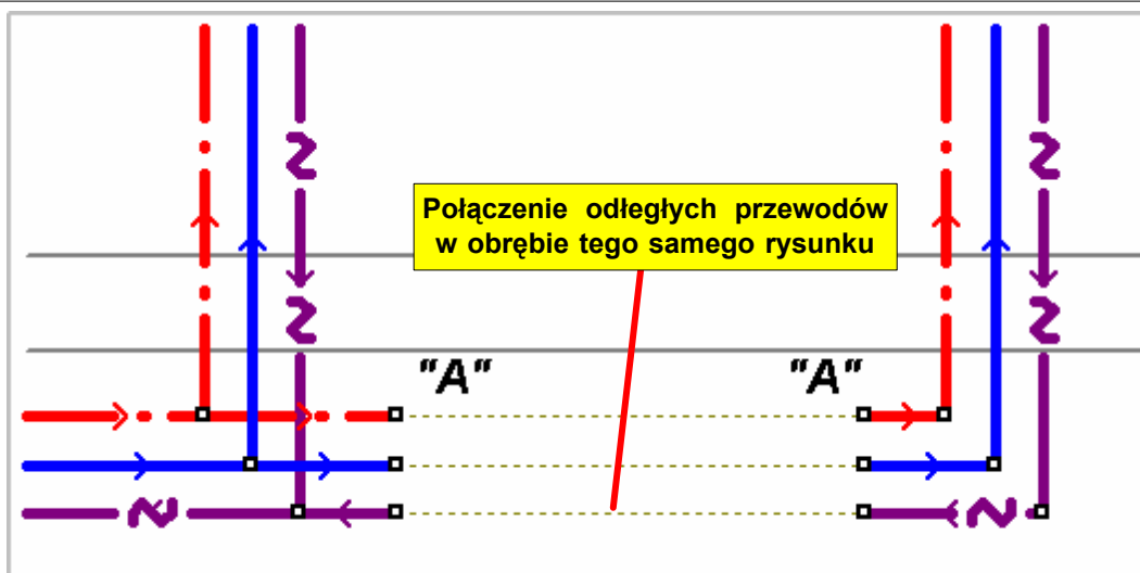
Połączenie odległych przewodów w obrębie rysunku
