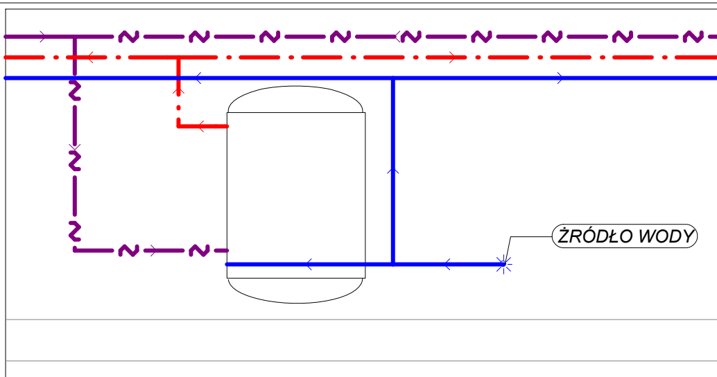
Fragment instalacji z zasobnikiem ciepłej wody
