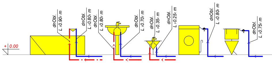
Elementy instalacji w łazience w systemie rozdzielaczowym
