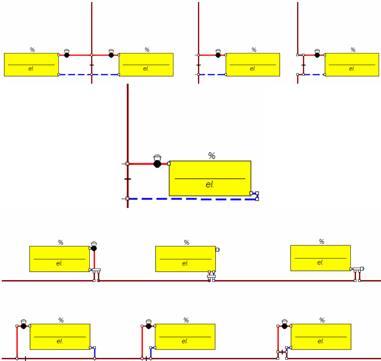
Przykłady podłączenia grzejników w instalacji jednorurowej
