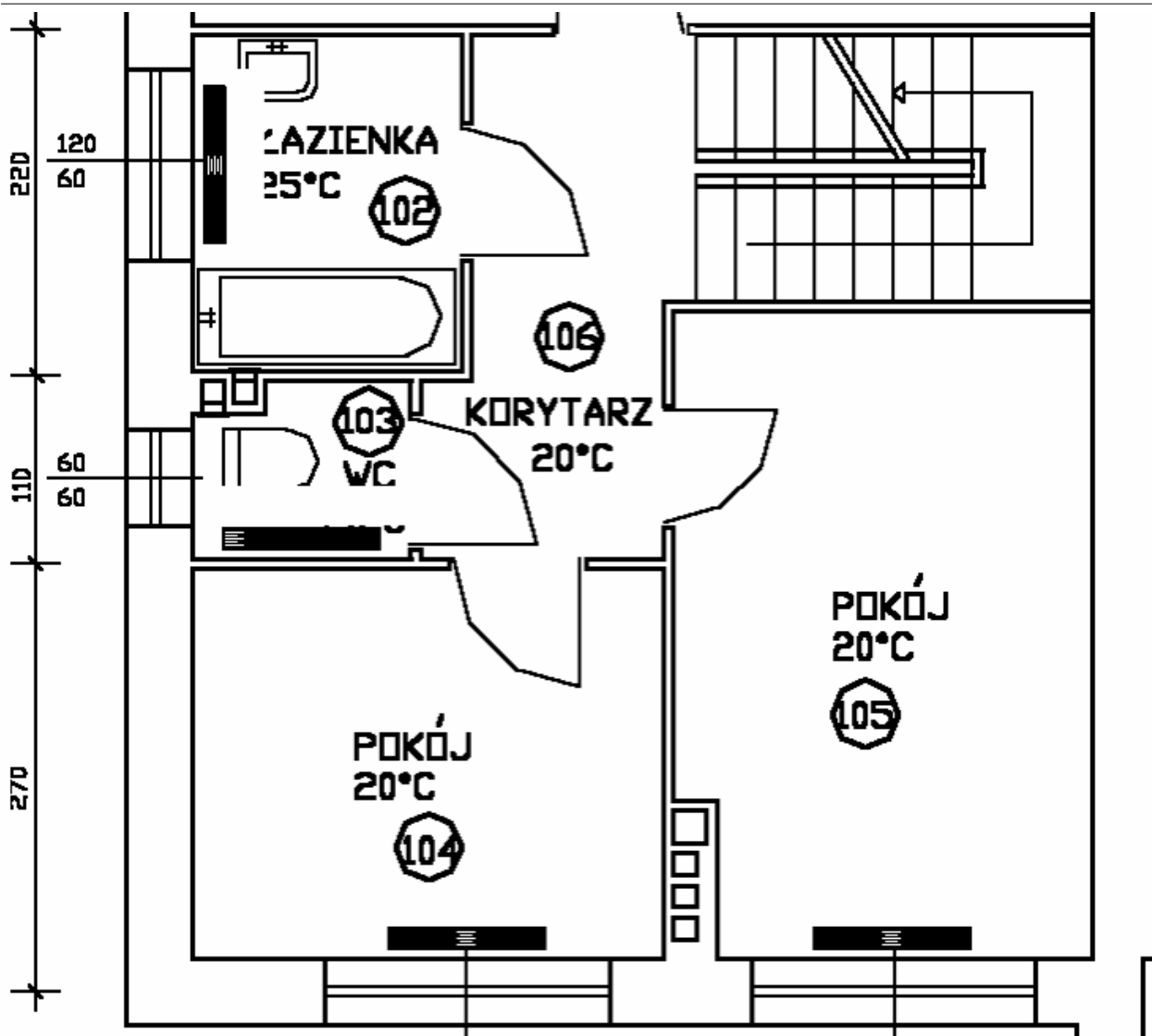
Rzut z naniesionymi i powiązаныmi grzejnikami konwekcyjnymi
