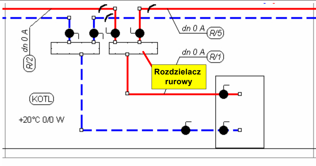
Fragm. rysunku ze źródłem ciepła i siecią przewodów rozprowadzających, armaturą odcinającą, strefą pomieszczenia oraz etykietami przewodów
