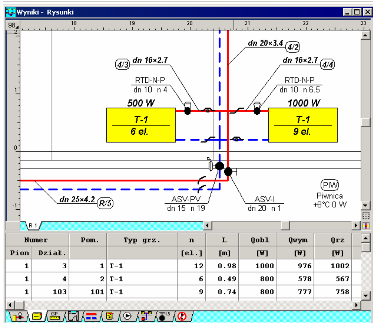
Fragment rozwinięcia z wynikami obliczeń
