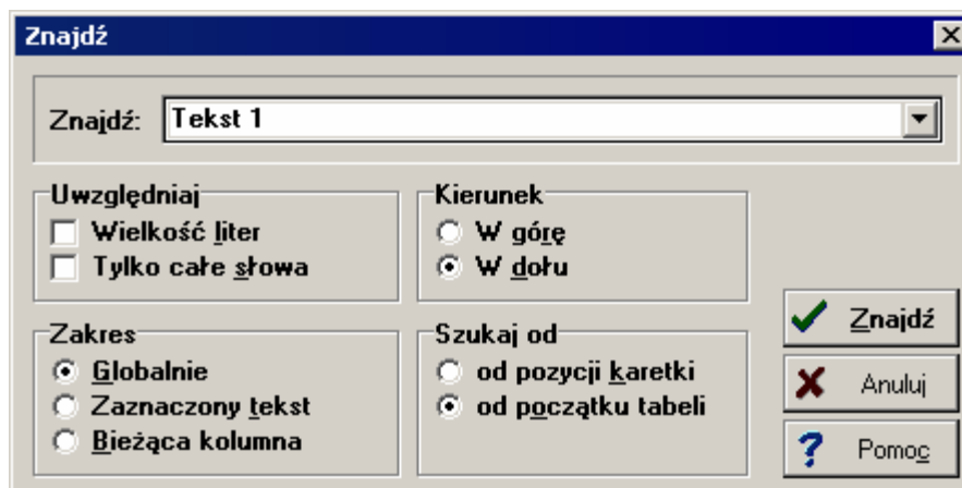
Dialog Znajdź
