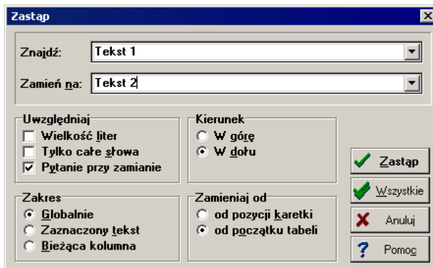
Dialog Zastąp
