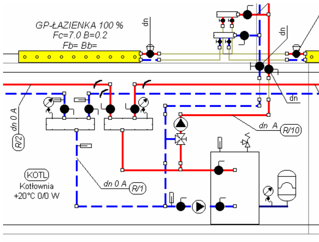
Fragment rysunku ze źródłem ciepła i siecią przewodów z narysowanymi termometrami, pompą i zaworem bezpieczeństwa
