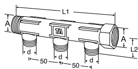
TA 56 043, Rozdzielacz 3-obwodowy Z nakrętką
